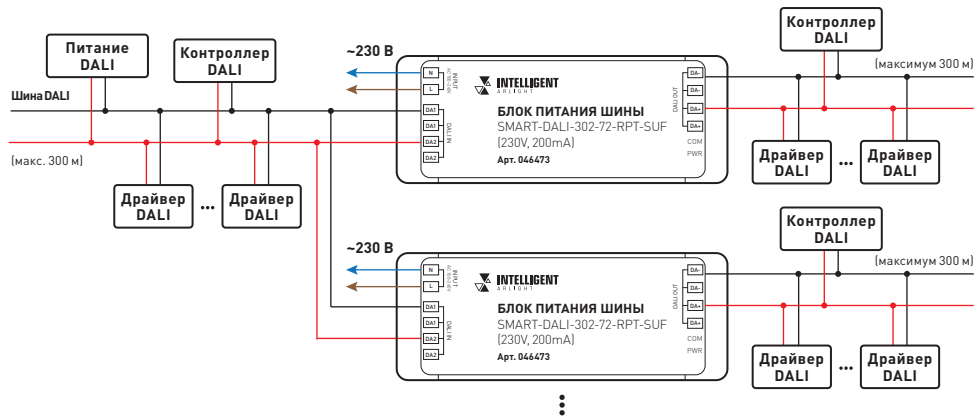
Рис. 3. Схема подключения шины DALI вертикальное размещение
