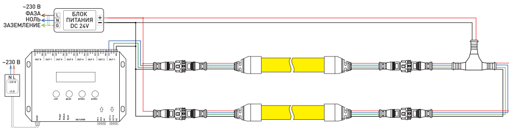
Рис. 1. Схема подключения питания с обеих сторон неона и с использованием одного источника напряжения
