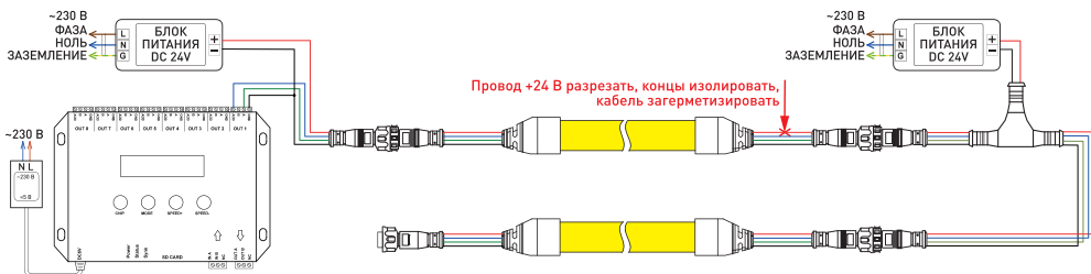
Рис. 2. Схема подключения питания с использованием двух источников напряжения
