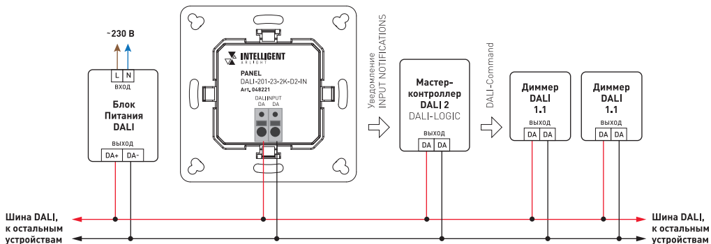
Рис. 1. Пример схемы подключения панели
