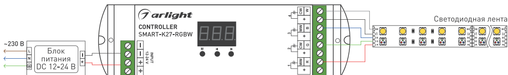
Рисунок 1. Схема подключения контроллера SMART-K27-RGBW
