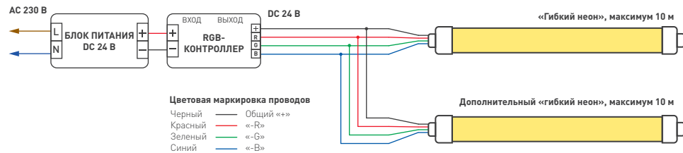
Схема 1. Подключение герметичной ленты «неон»
