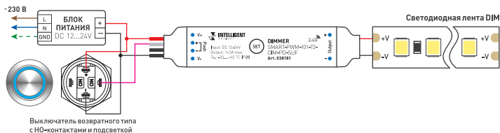
Рис. 2. Схема подключения диммера с использованием кнопки с подсветкой
