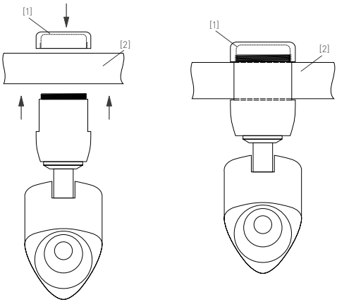
Рис. 2. Установка светильника
