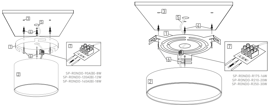
Рис. 2. Установка и подключение светильника
