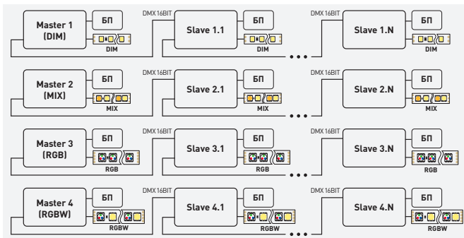
Рис. 2. Общая структурная схема построения системы управления освещением
