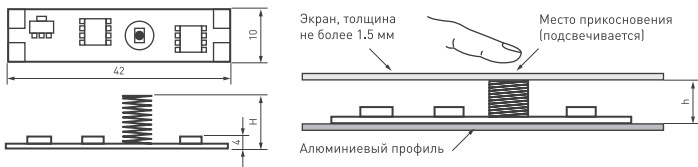
Рисунок 1. Установка микродиммера.
